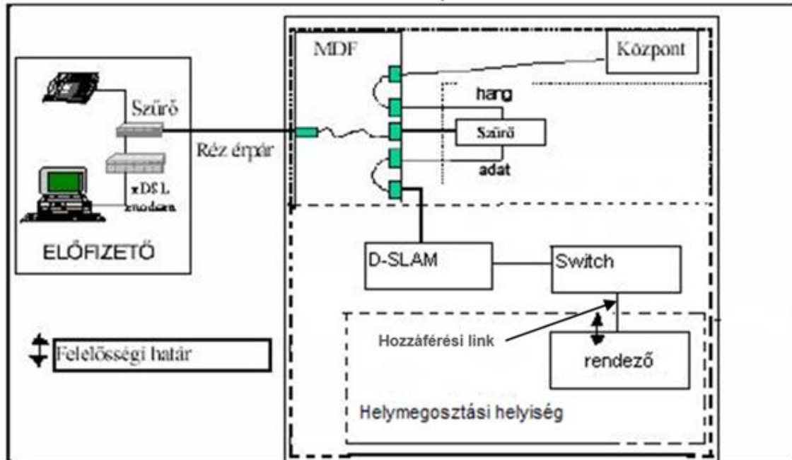
Közelit bitfolyam hozzáférés réz érpáras hálózaton, helymegosztás esetén
